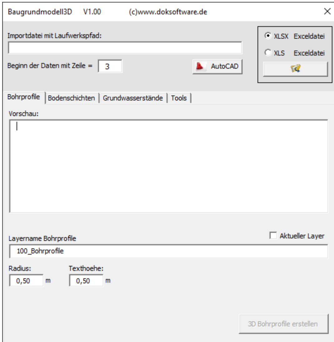
Bild 2: Programmoberfläche
